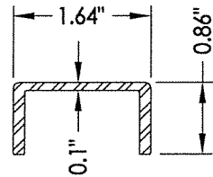
22 REINFORCEMENT 356-A61-A
